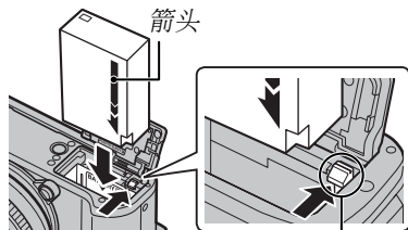
电池释放搭扣
