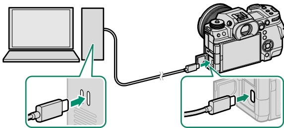
USB-aansluiting (Type-C)
