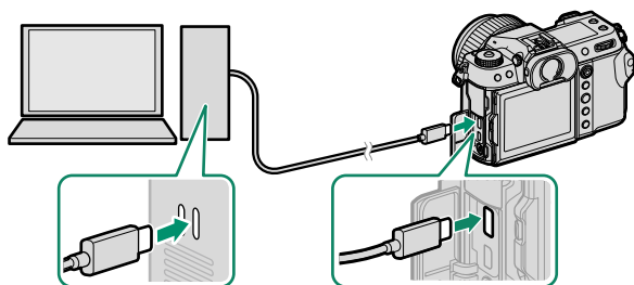
USB-aansluiting (Type-C)
